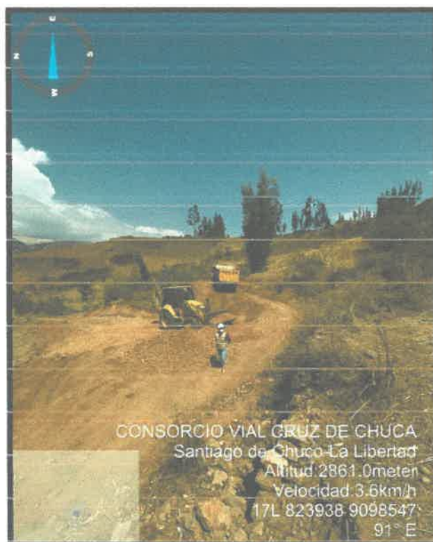
Foto N°02: Verificación de material insitu en la vía a ejecutar.
