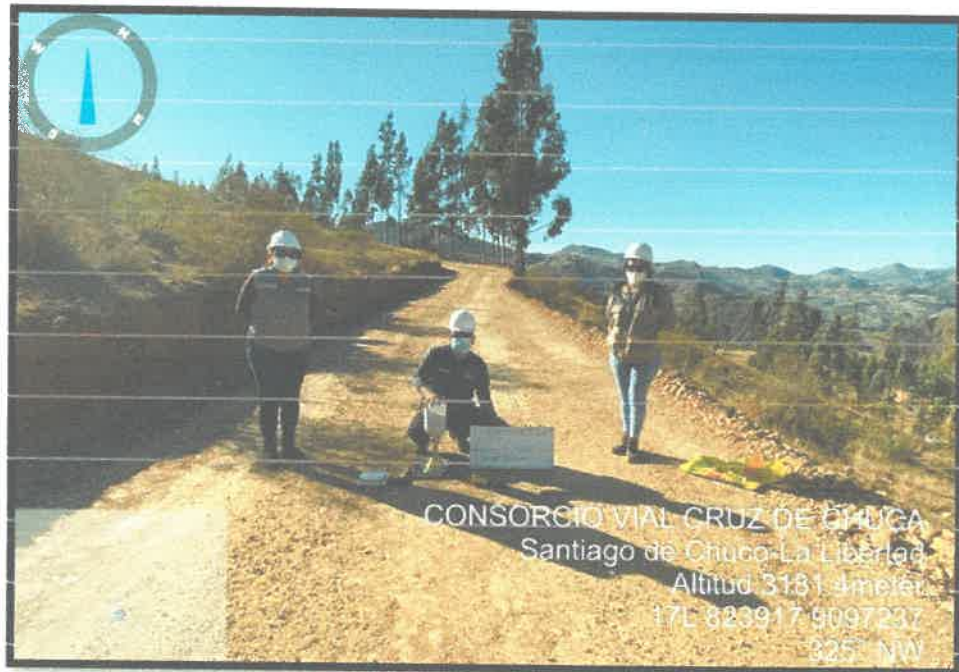
Foto N°05: Presencia de la Ing. Residente con la ing. Inspectora realizando los respectivos controles de calidad del afirmado (densidad de campo)
