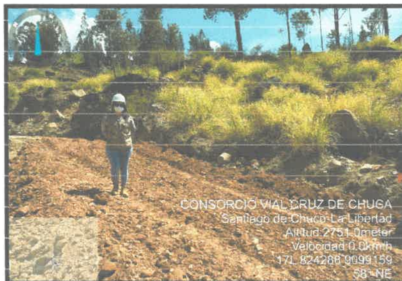
Foto N°01: Conformación de plataforma con espesor de 0.20cm, punto crítico en el km 1+100 Sector El Ingenio.
