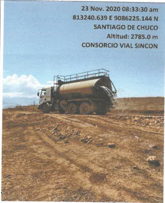
Proceso constructivo, Riego de la plataforma en el , km 25+000 9086225N 813240E
