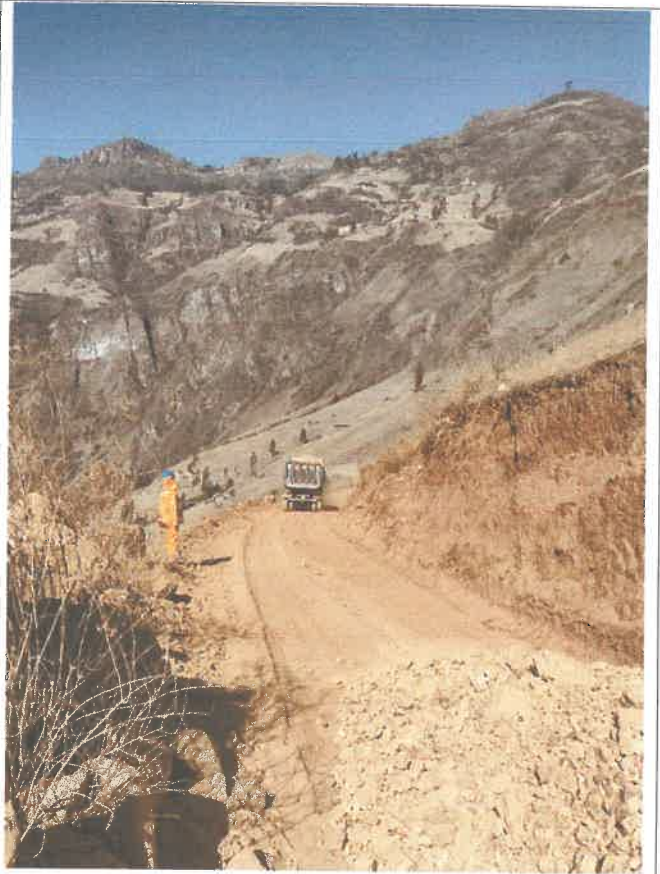
Verificación del proceso constructivo, colocación de capa nivelante e=0.05m , Km 23+500, 9082444N 806233E
