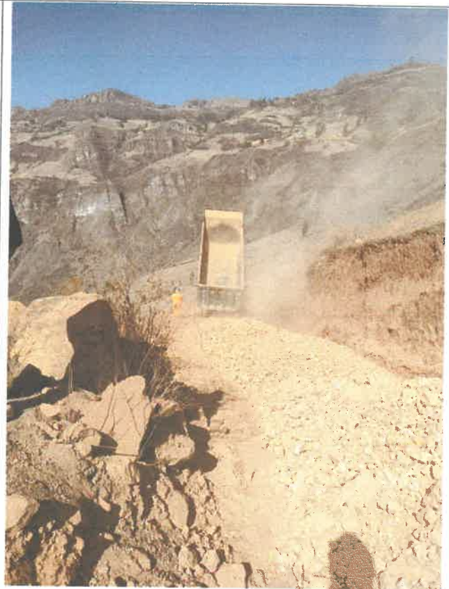
Colocación de material granular de cantera e=0.15m, km 17+500 9089954N 813813E
