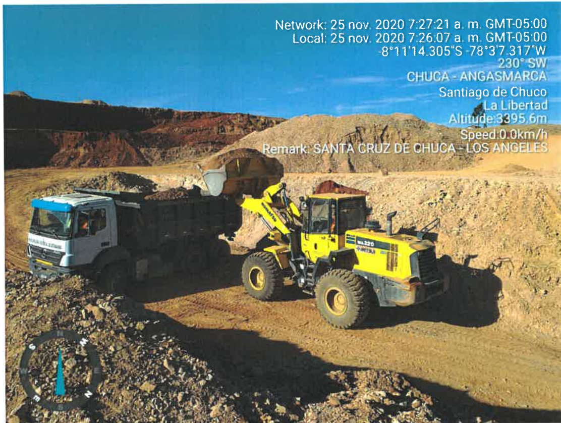
Foto N° 05: Se observan el acopio en cantera de material granular hasta 1km
