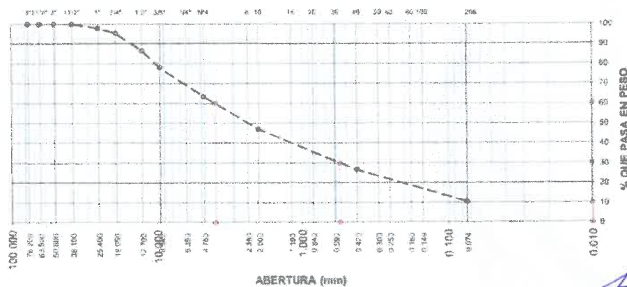
CURVA GRANULOMETRICA
