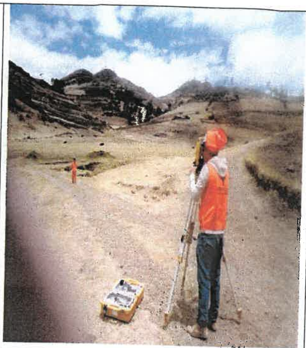
Trazos y replanteos referidas al tramo 13, entre las localidades de Caypanda – casa de calamina - Imball 9088824 N 810165 E
